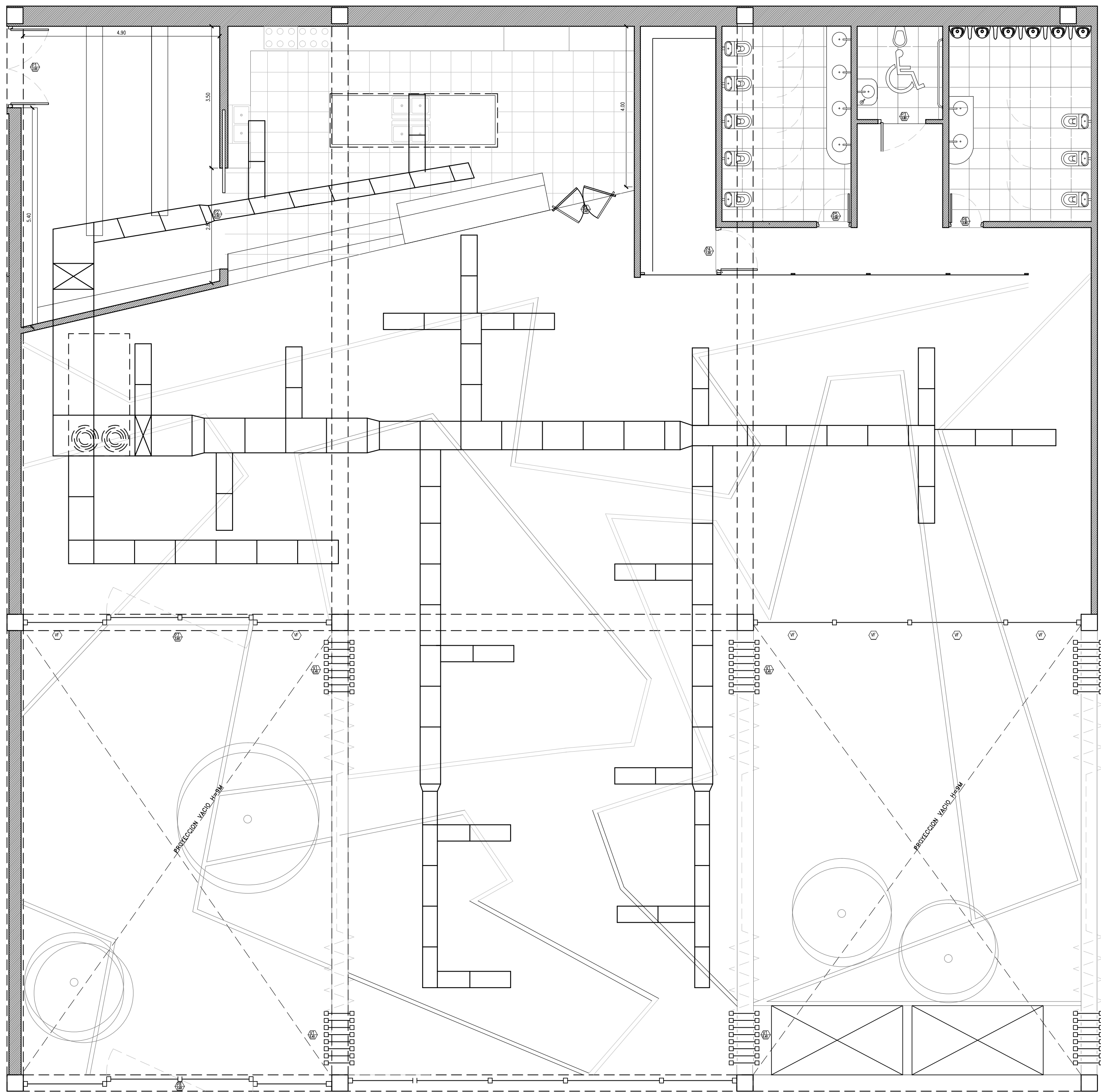
PLANTA BAR - Conducto Aire acondicionado
