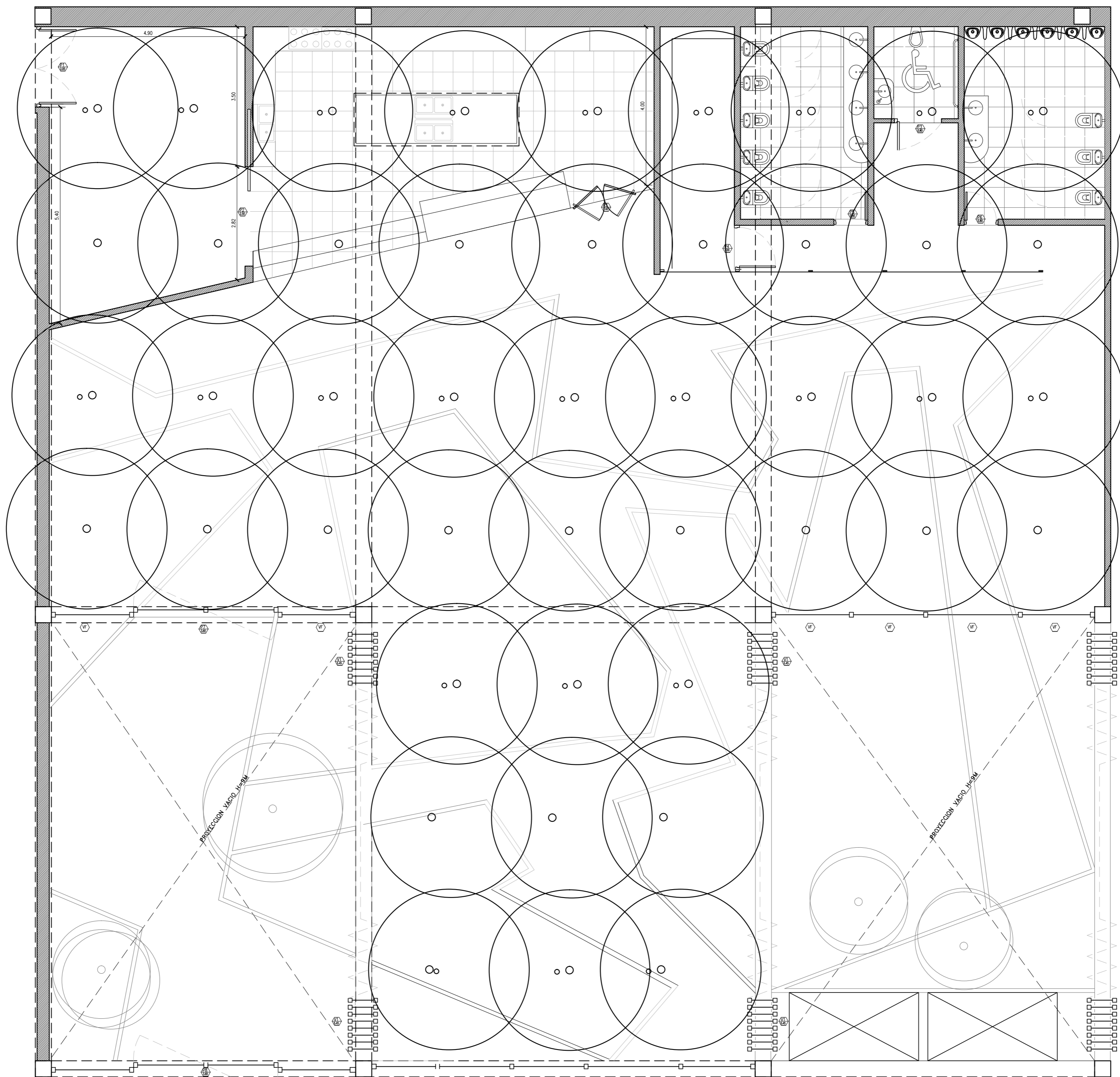
PLANTA BAR - Aspersores / Detectores de humo
