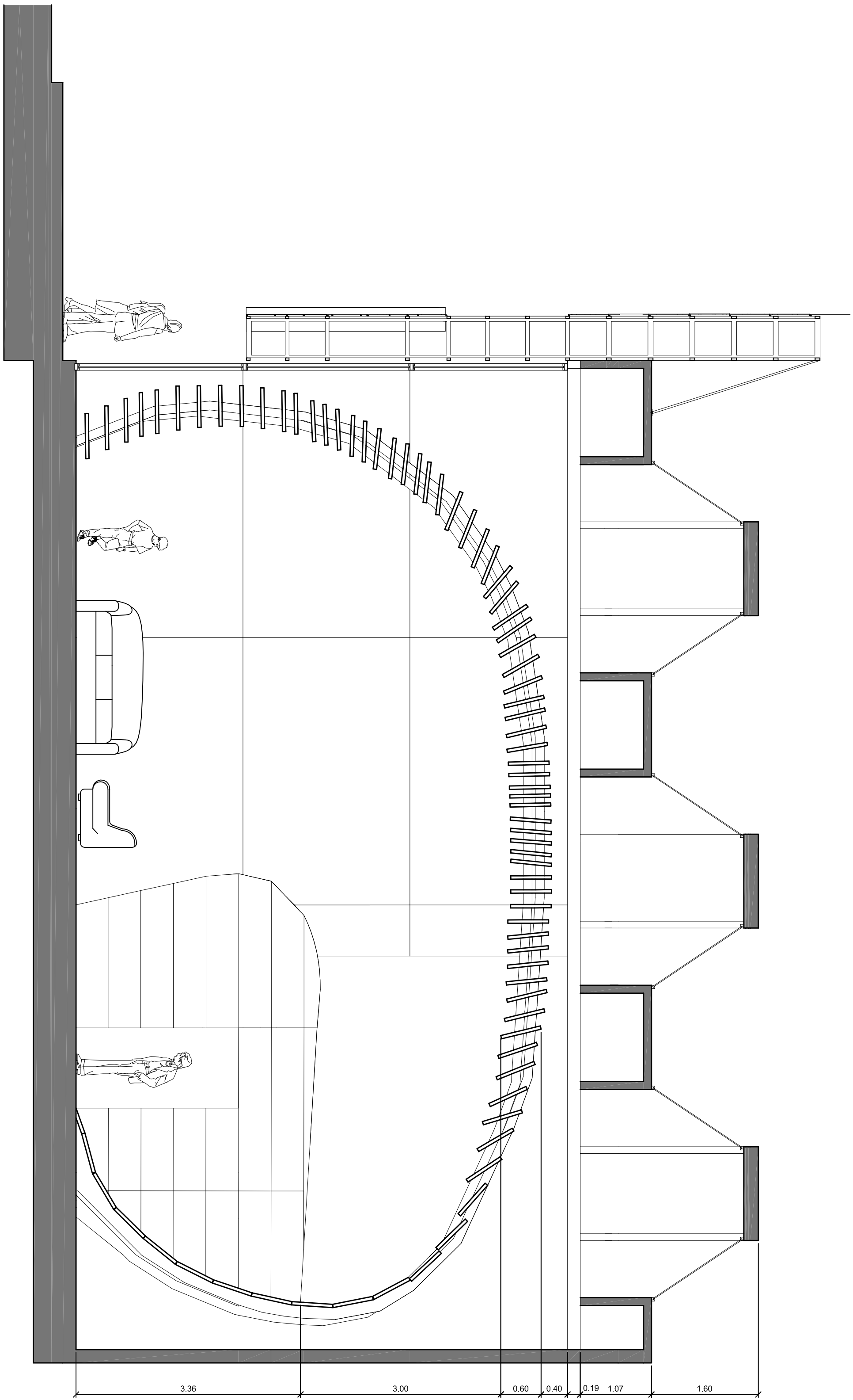
CORTE A-A ESC. 1:50
